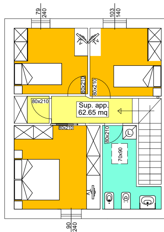
PIANO PRIMO
