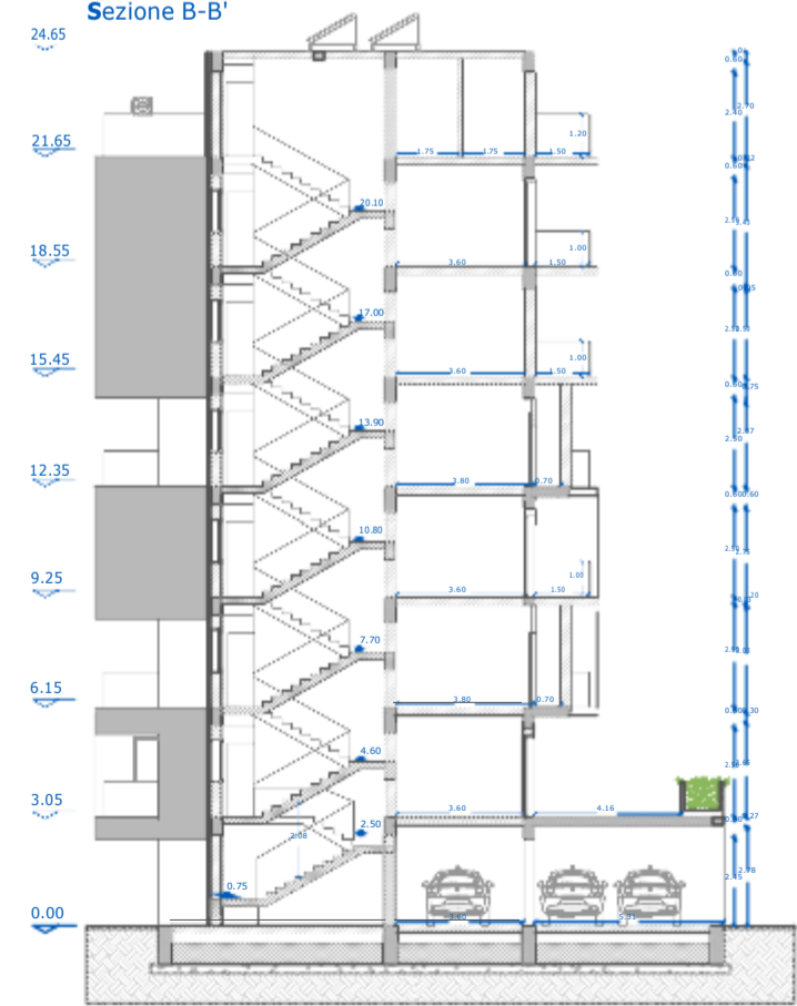
Stato di Progetto Sezione B-B'
