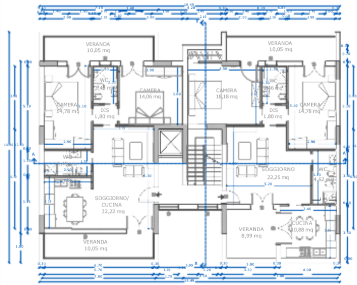
Stato di Progetto Pianta Piano Quarto
