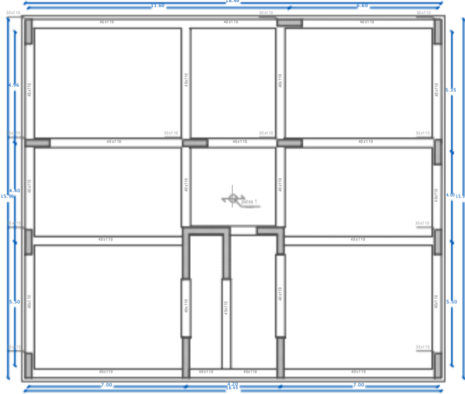
Stato di Progetto Pianta Piano Quarto
