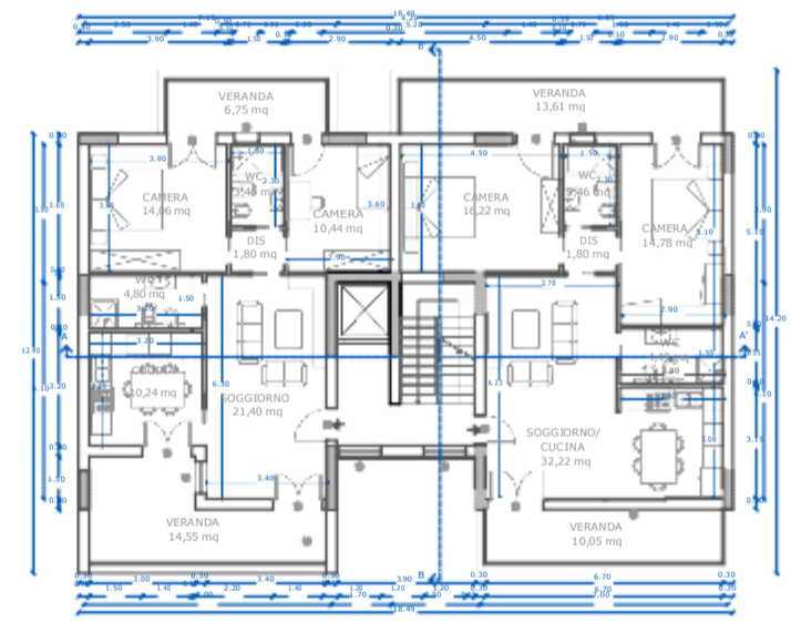
Stato di Progetto Pianta Piano Quinto
