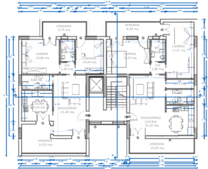
Stato di Progetto Pianta Piano Sesto
