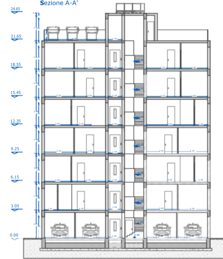
Stato di Progetto Sezione A-A'
