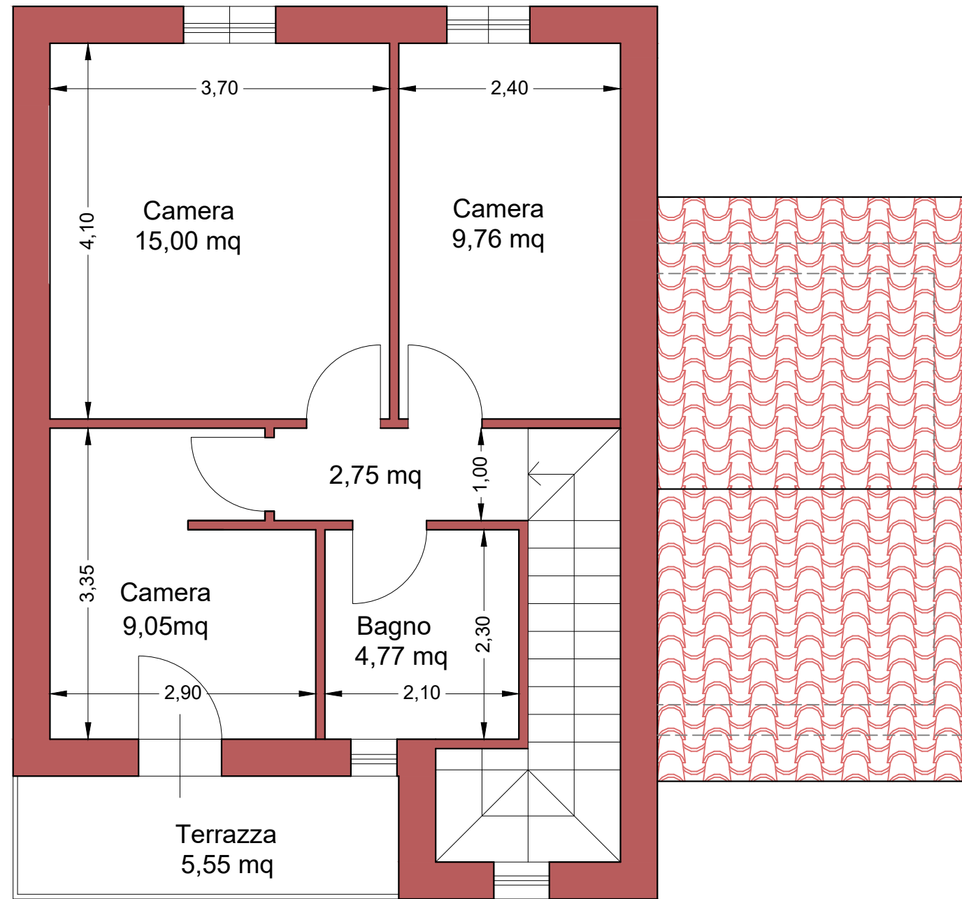
PIANO PRIMO
