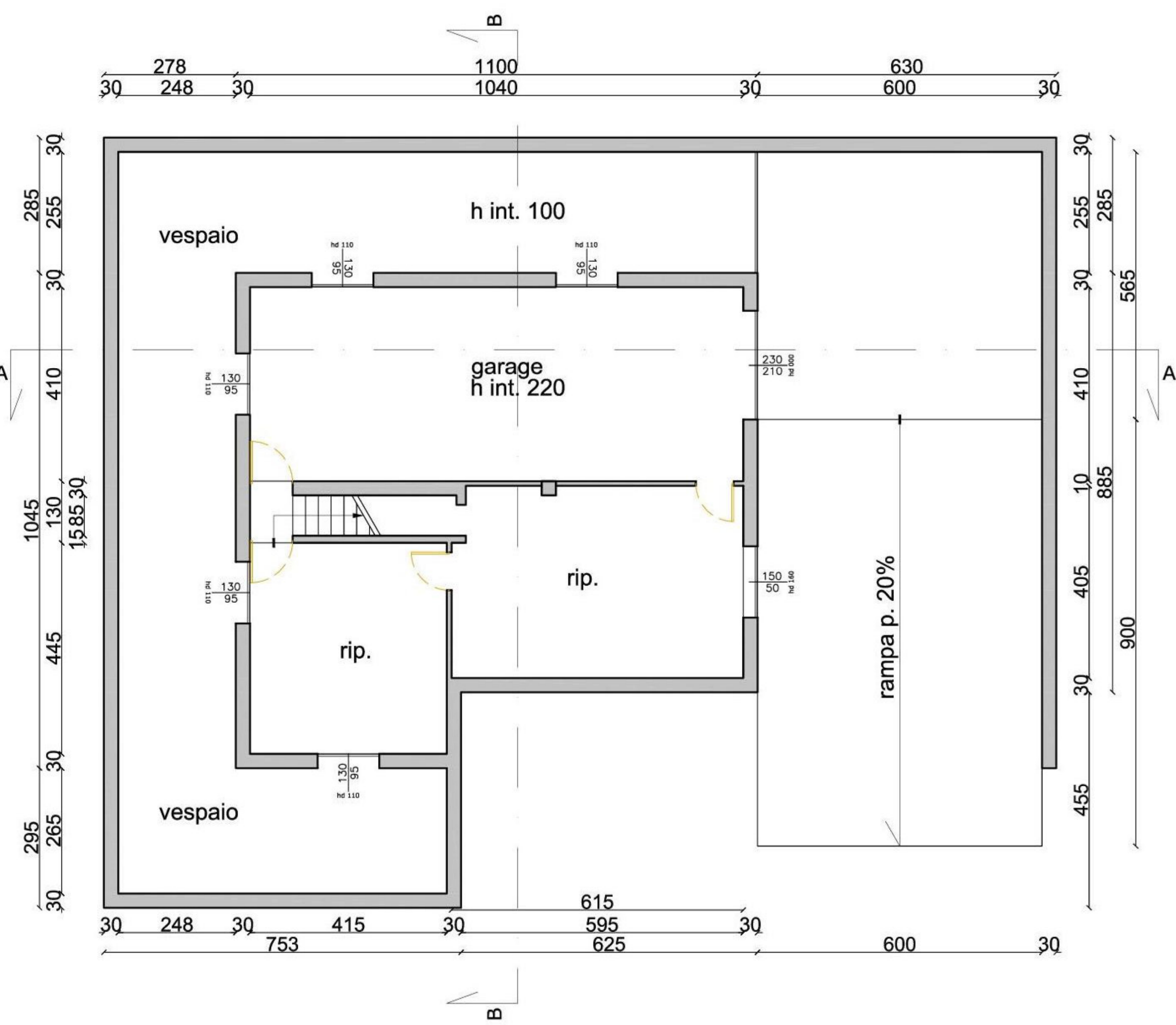
PIANTA PIANO INTERRATO
