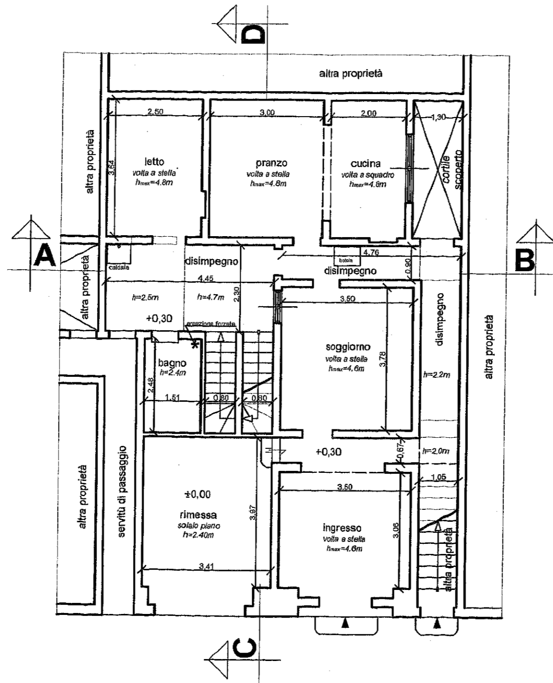
piano terra ( progetto )
