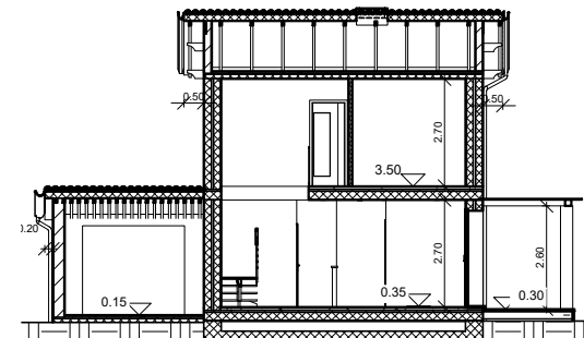
SEZIONE B-B
