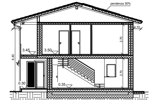
SEZIONE A-A
