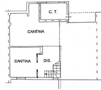
PIANO PRIMO SOTTOSTRADA H.=2.08ml.
