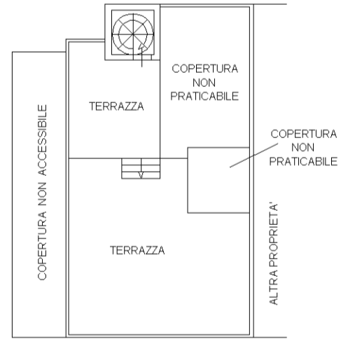
PIANO TERZO (COPERTURA)
