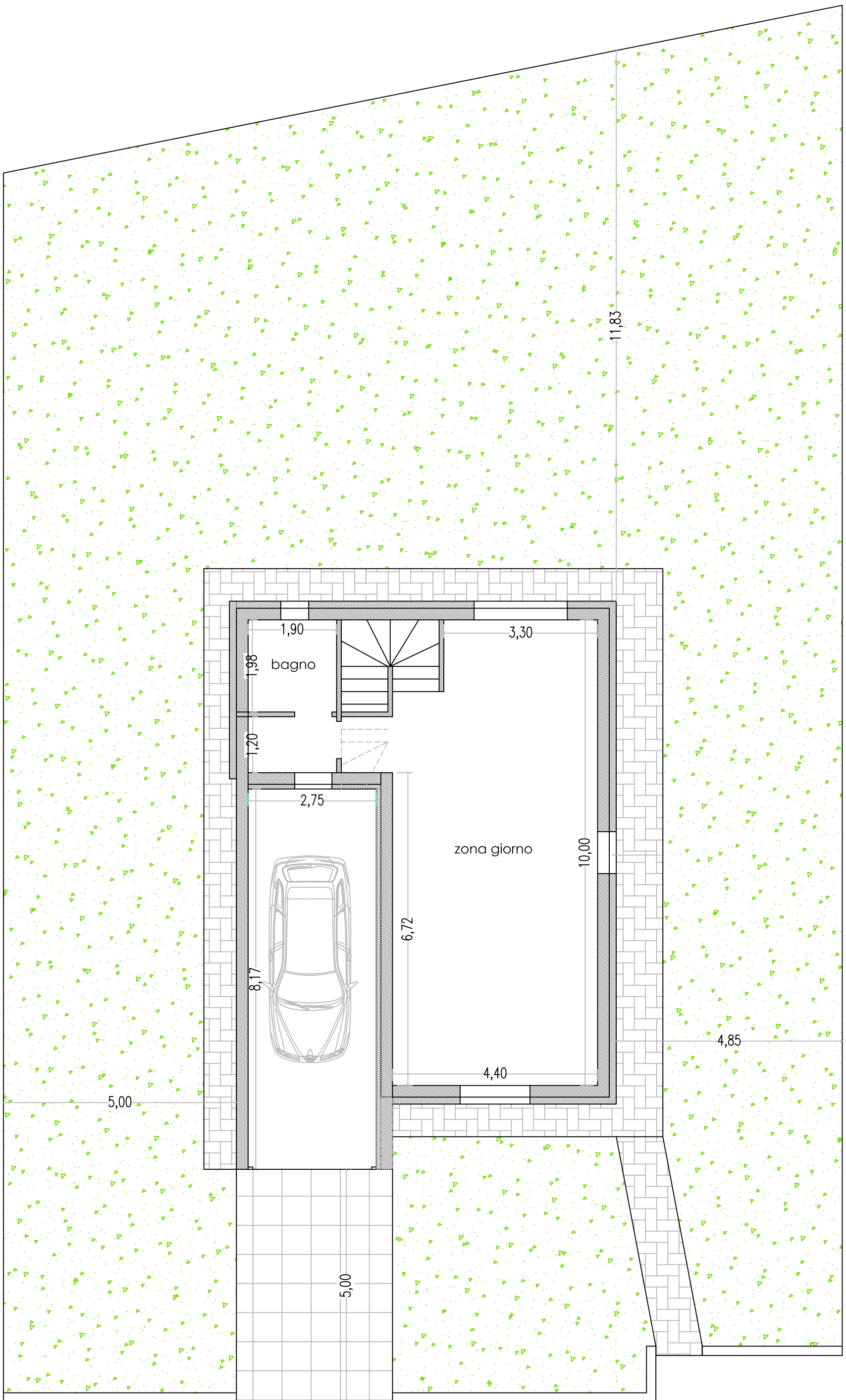
PLANIMETRIA - pianta PIANO TERRA
