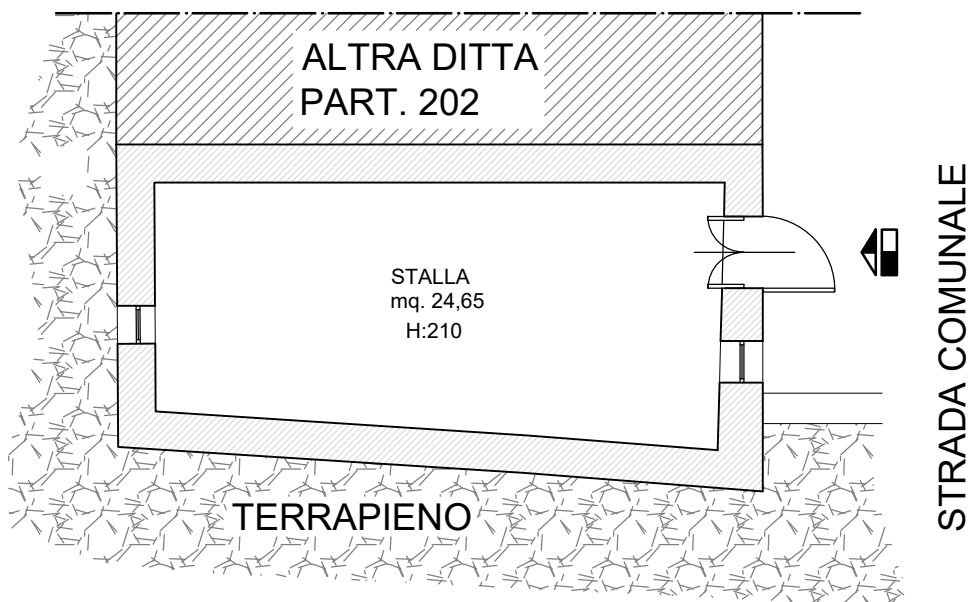
Pianta Piano Seminterrato
