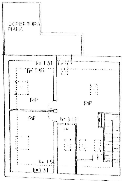
PIANO SECONDO SOTTOTETTO
