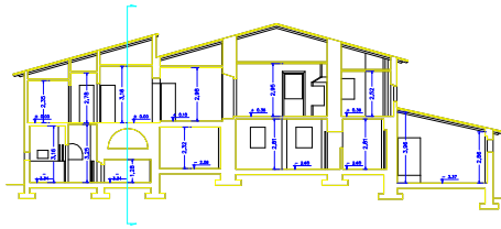
SEZIONE A-A' scala 1:100
