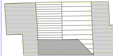
PIANTA DELLE COPERTURE scala 1:100
