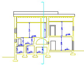
SEZIONE A-A' scala 1:100
