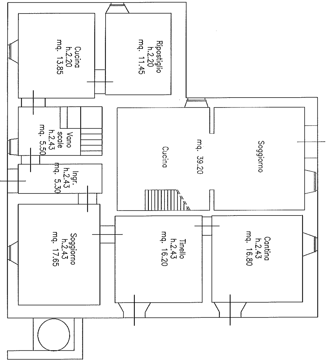
PIANTA PIANO TERRA SUPERFICIE COMMERCIALE MQ. 189.00
