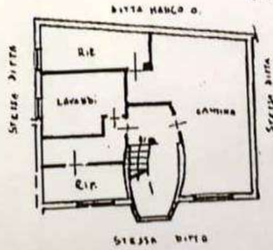
PIANO SEMINTERRATO m. 2,60
