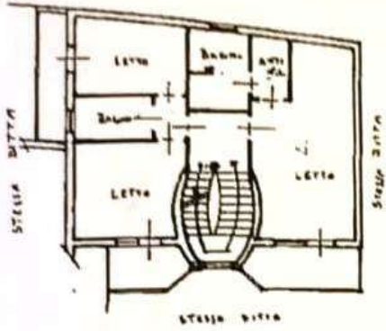
PIANO PRIMO m. 2,95
