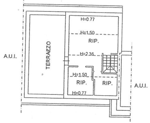
PIANO SOTTOTETTO H=2.70m
