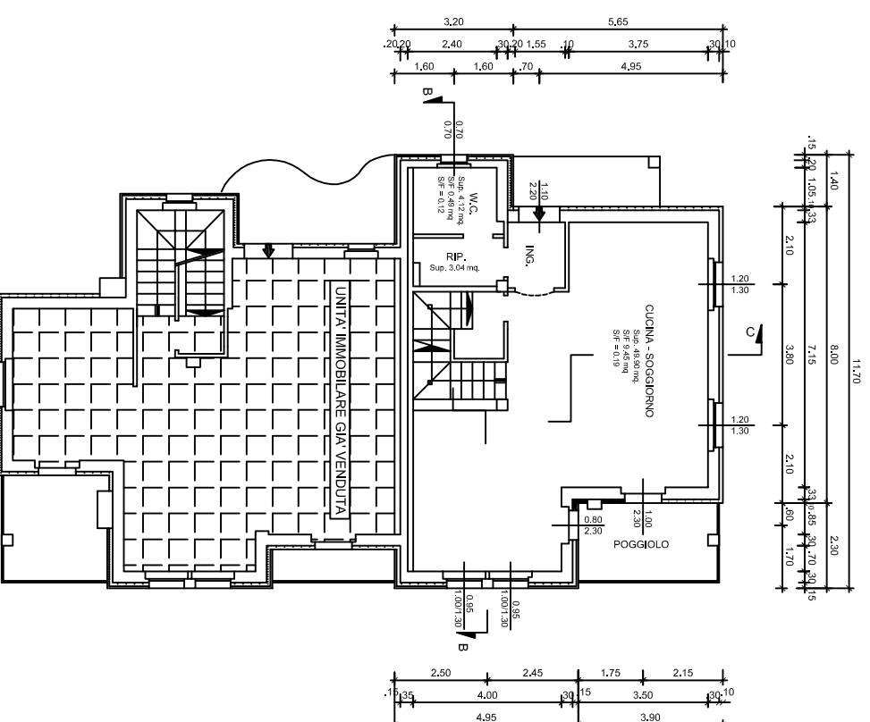
PIANO TERRA-RIALZATO
