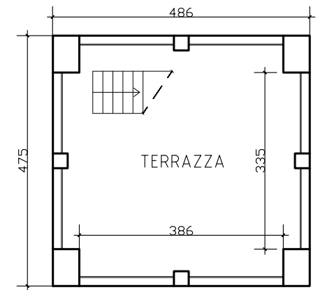
PIANTA PIANO QUARTO (COPERTURA) S.U.L. mq. 23,09 scala 1/100
