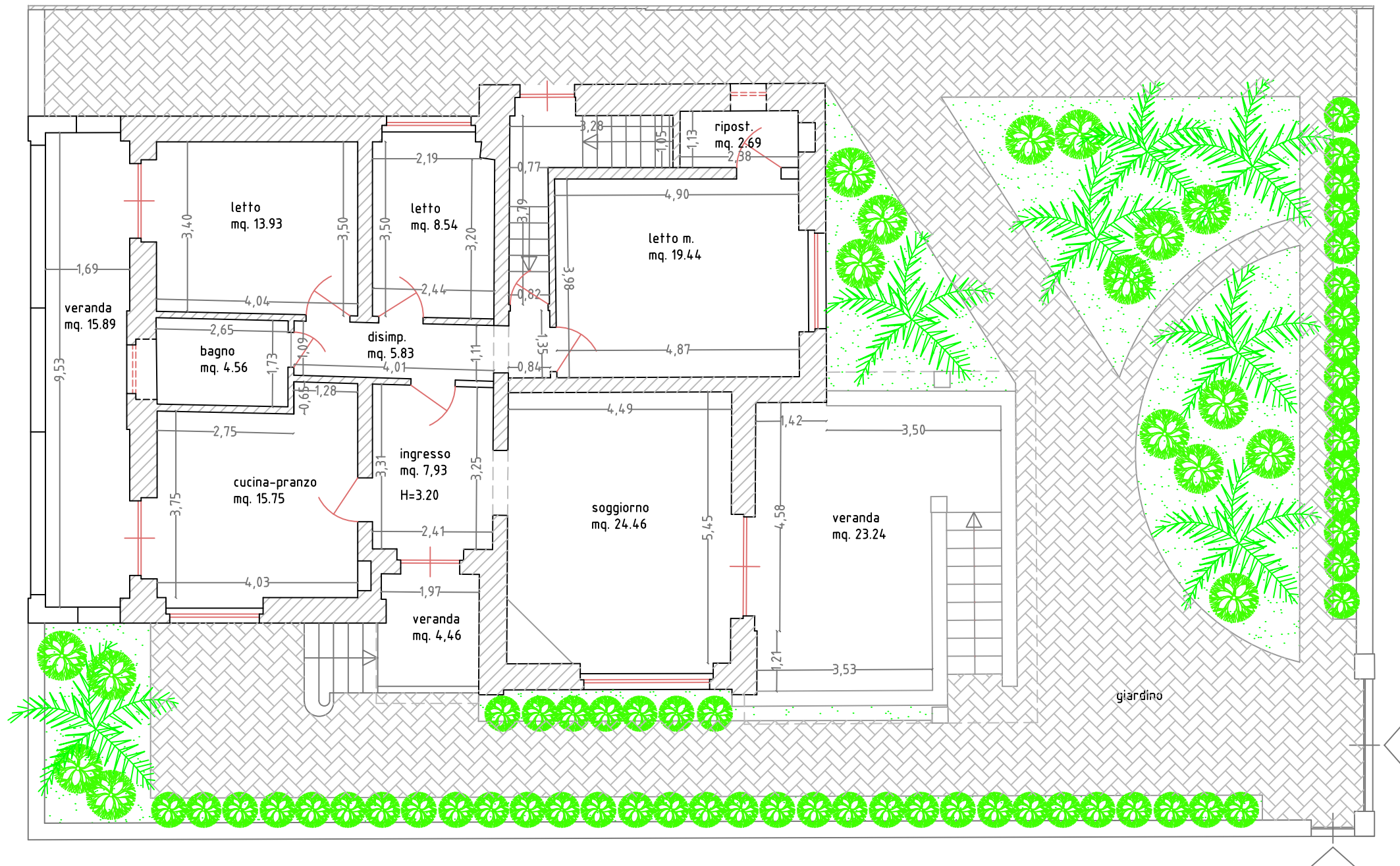
PIANTA PIANO RIALZATO rapp. 1:100
