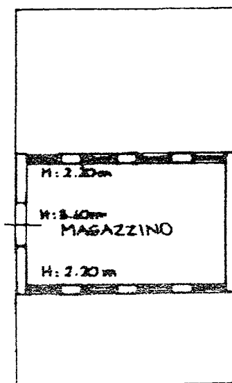
PIANO PRIMO
