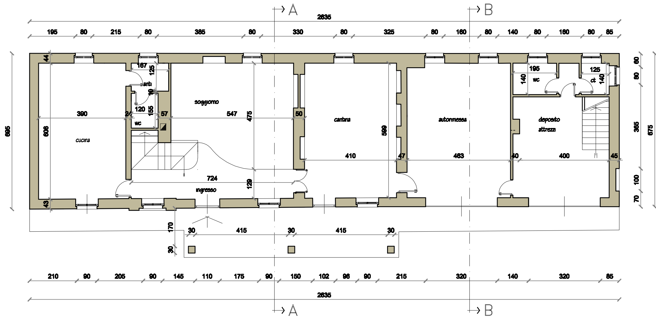
PIANTA PIANO TERRENO
