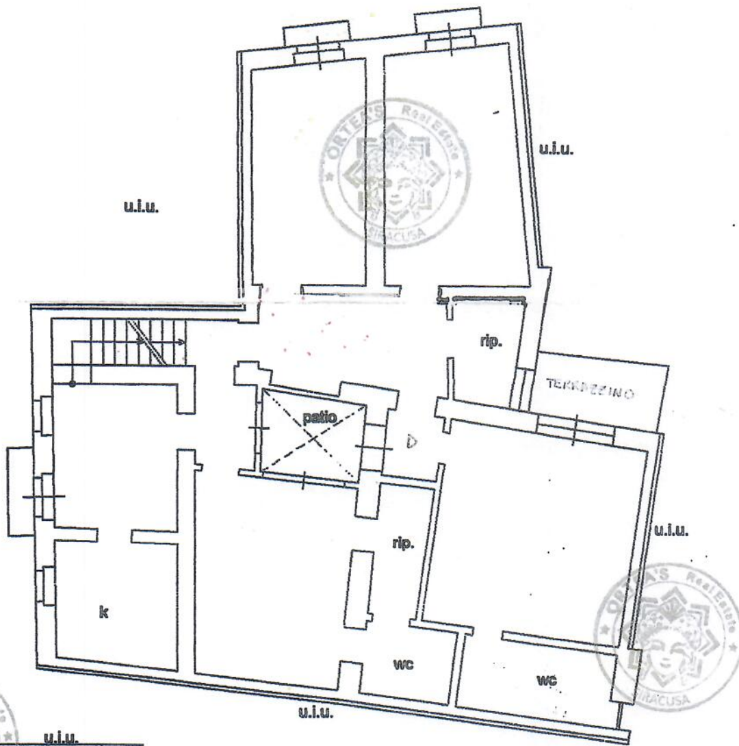
PIANTA PIANO PRIMO H=3,80m
