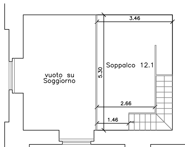
Planimetria soppalco appartamento 12 Sub_166 (scala 1:100 A3)
