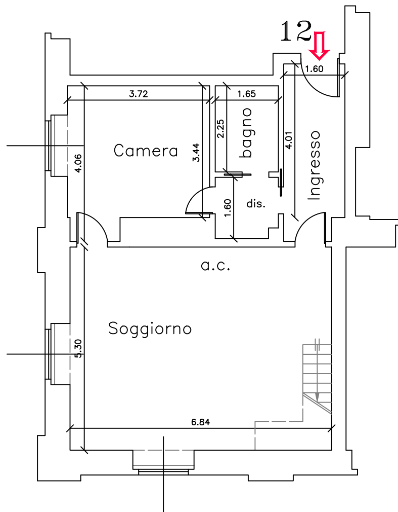
Planimetria appartamento 12 Sub_166 (scala 1:100 A3)
