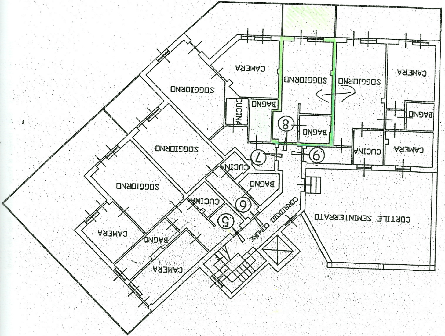
PIANTA PIANO PRIMO (2° F.T.) SCALA 1:200
