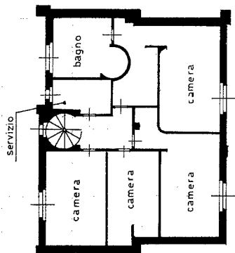
PIANO PRIMO HM. 270
