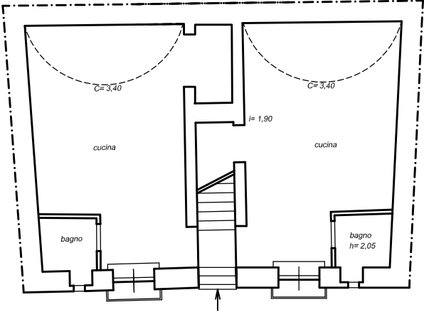
PIANO RIALZATO
