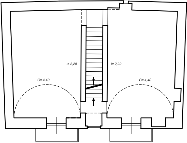
PIANO PRIMO
