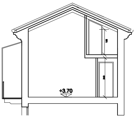
SOTTOTETTO U.I. 2 - SEZIONE 1-1
