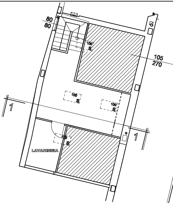
STRALCIO SOTTOTETTO U.I. 2
