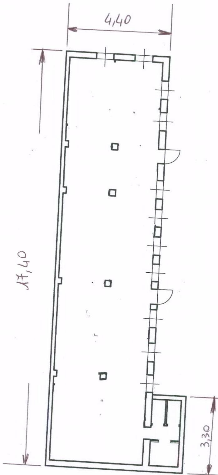
EDIFICIO 2 -demolizioni e costruzioni PIANO TERRENO - SCALA 1:100
