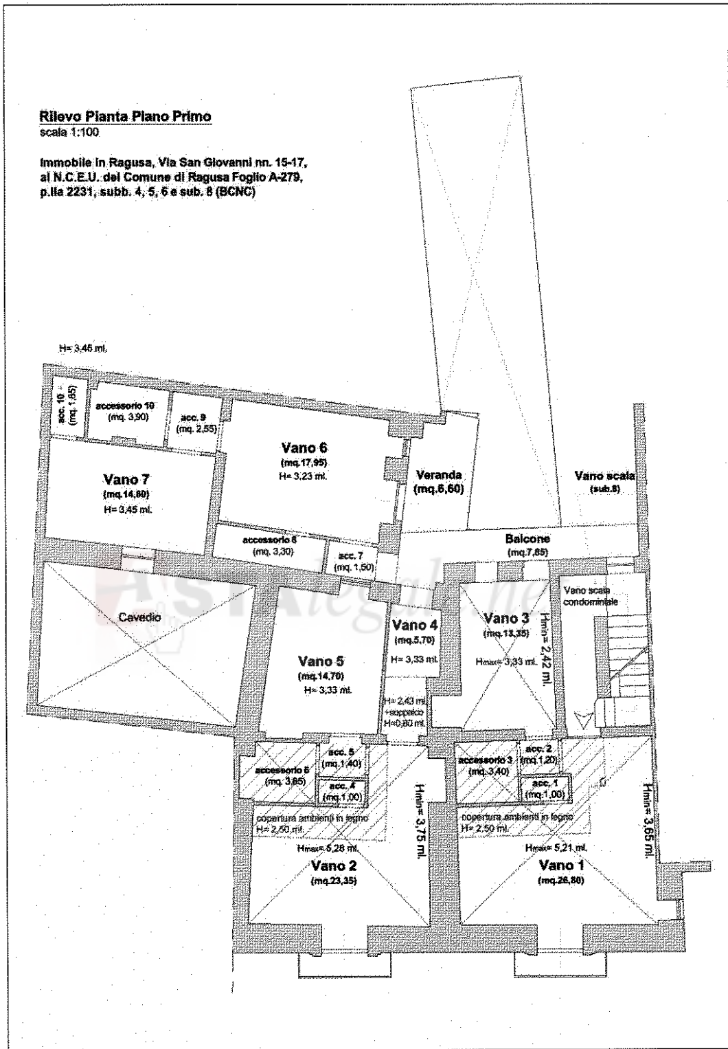
Rilievo Pianta Piano Primo
