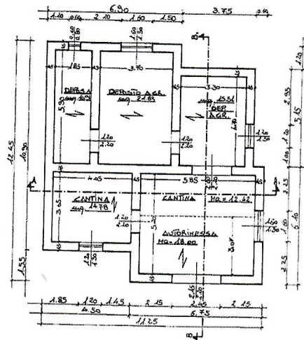
PIANTA PIANO TERRA Sc. 1:100
