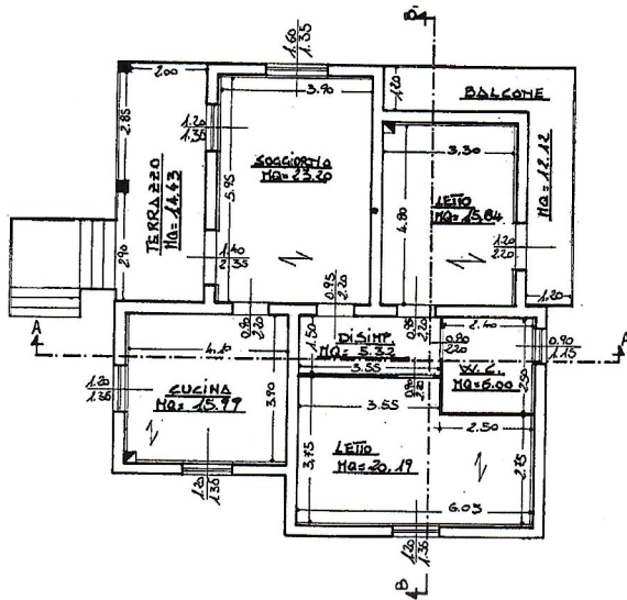
PIANTA PRIMO PIANO SCALA 1:100
