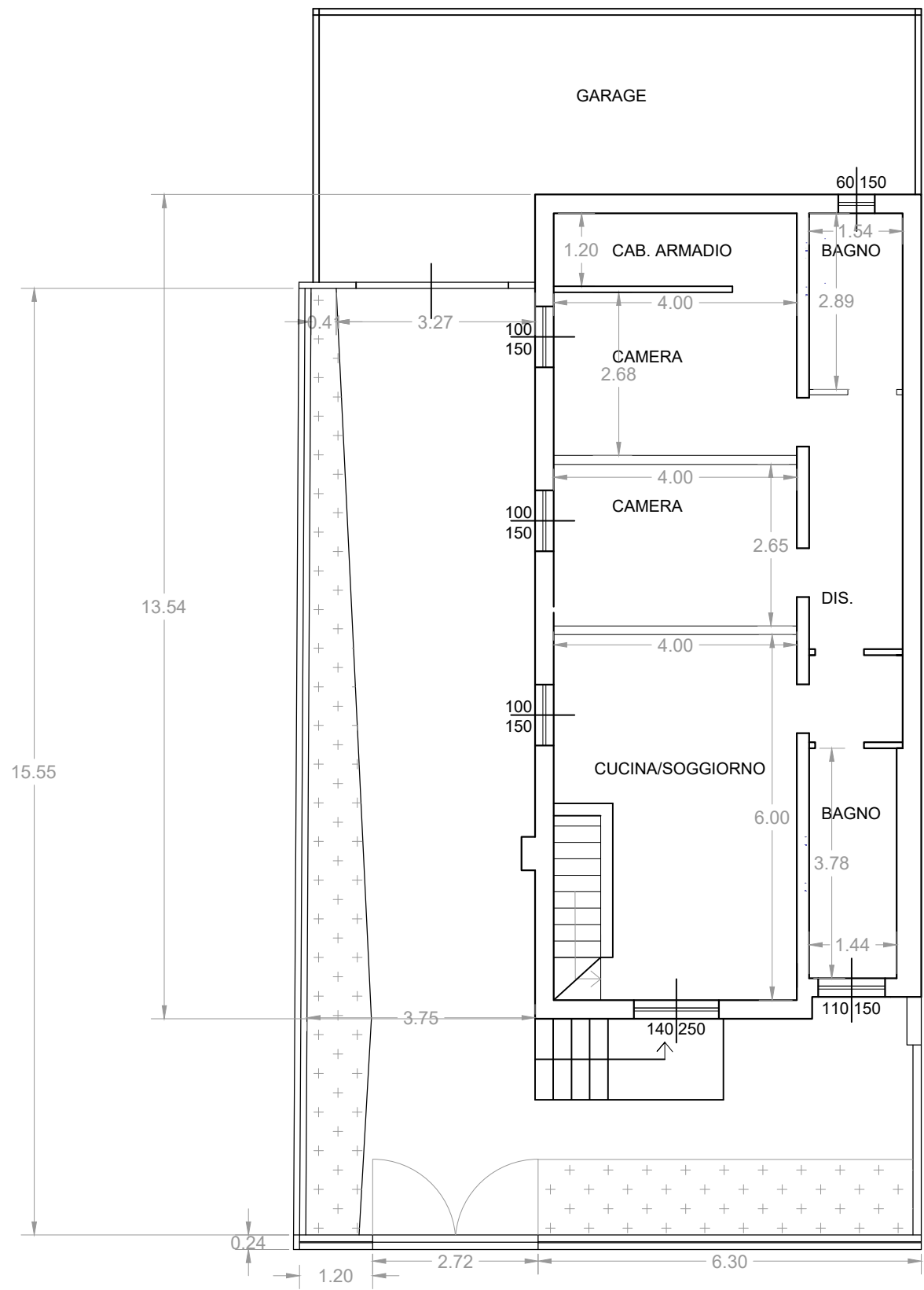
PIANTA PIANO RIALZATO RAPP. 1:100
