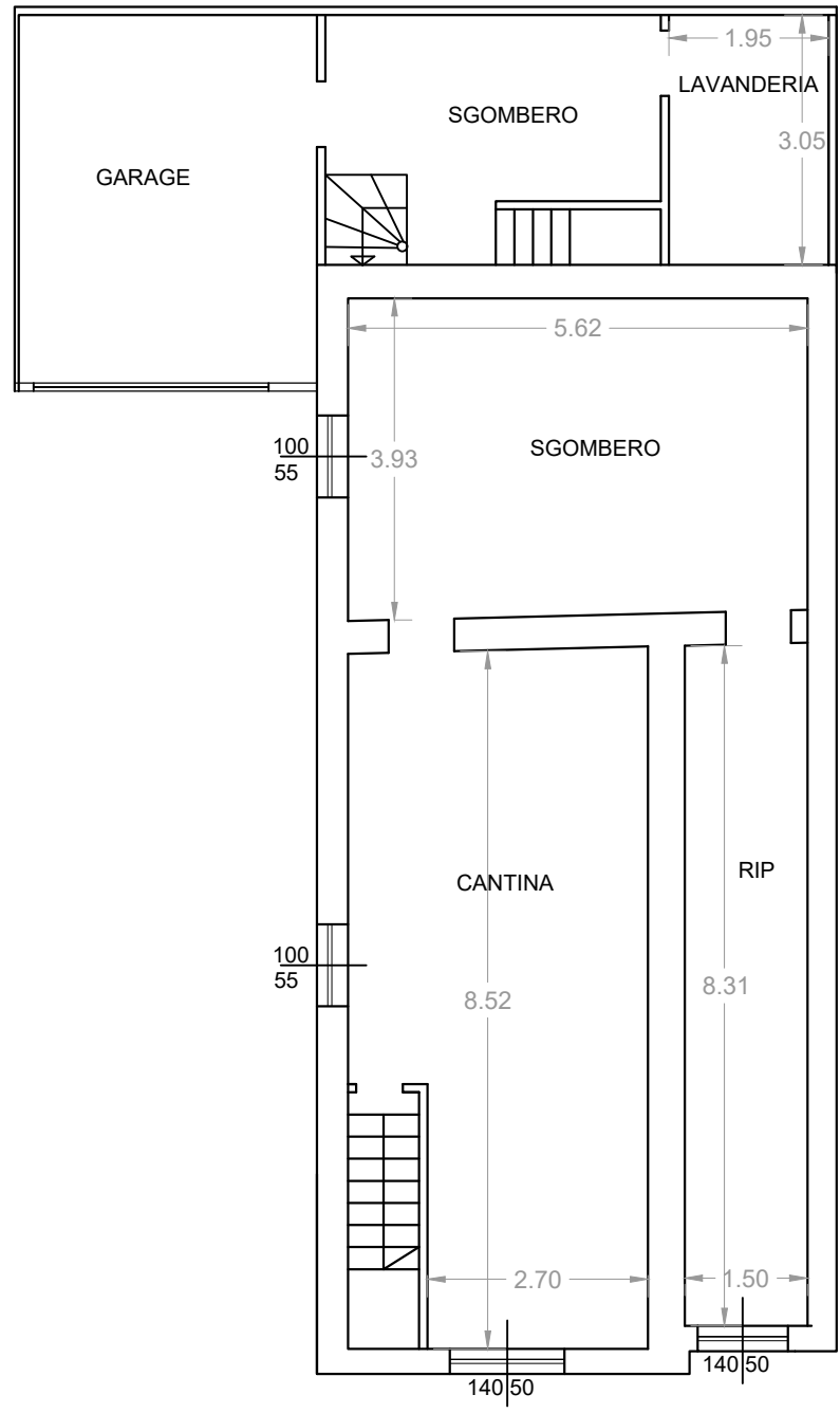
PIANTA PIANO SEMINTERRATO RAPP. 1:100
