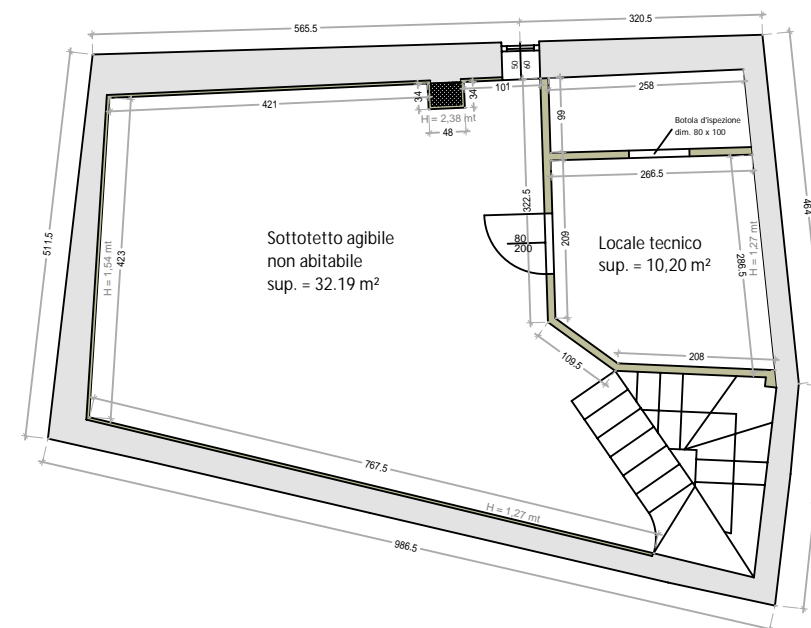
PIANTA SOTTOTETTO
