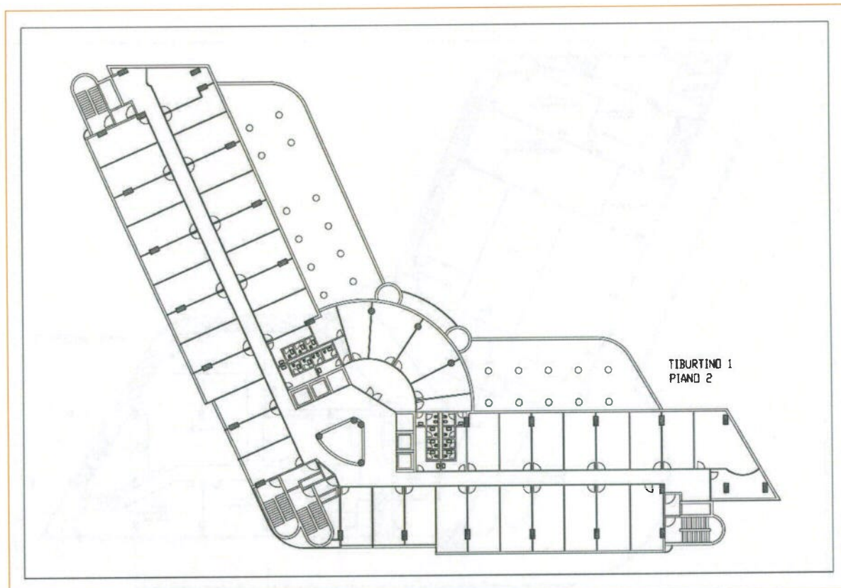
Planimetria Piano Tipo
