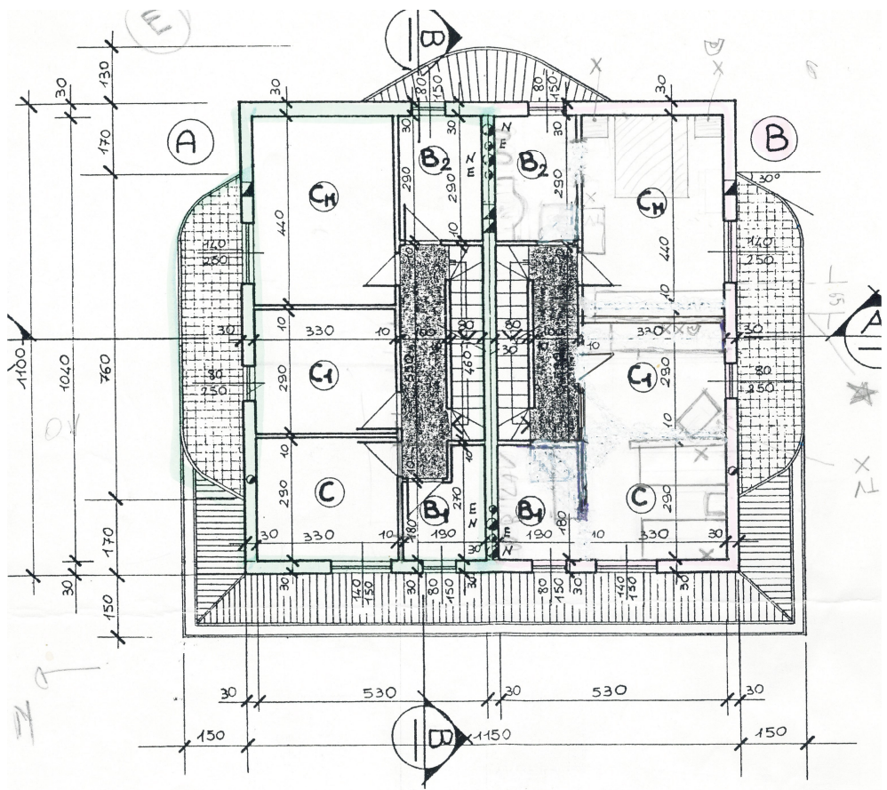
PIANO PRIMO
