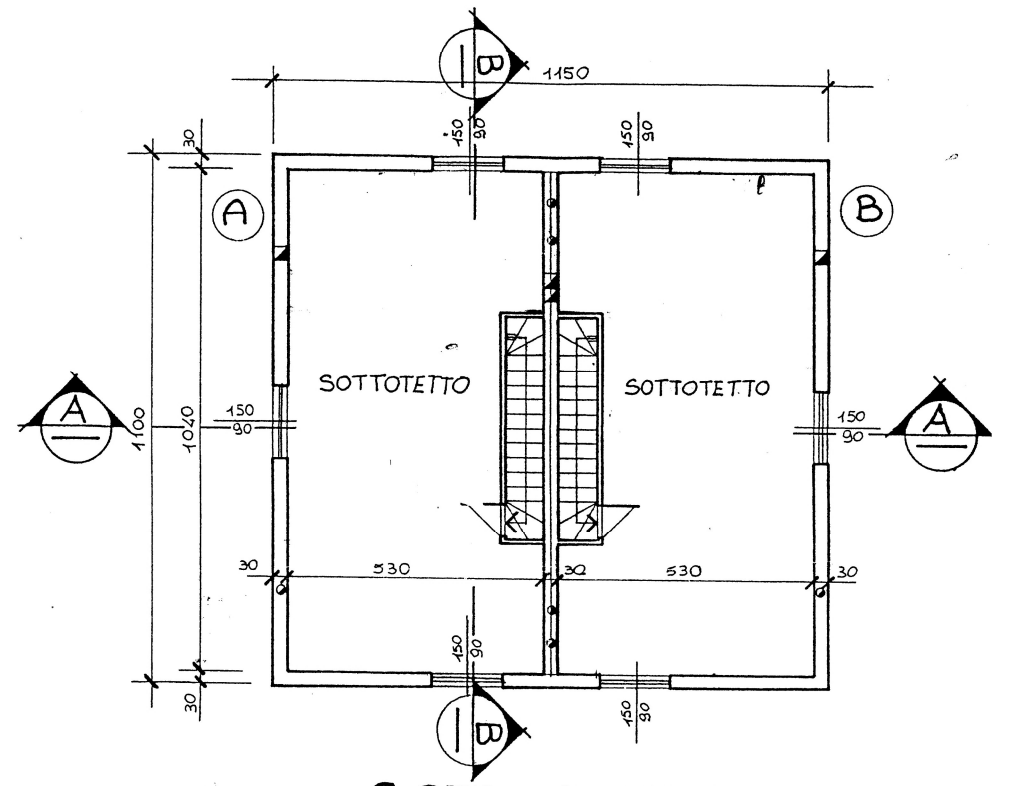
SOTTOTETTO
