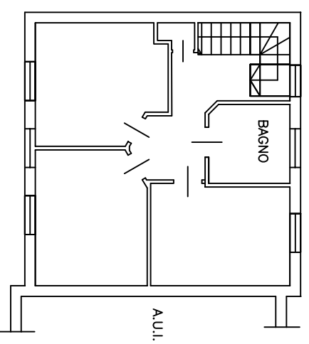
PIANO SECONDO
