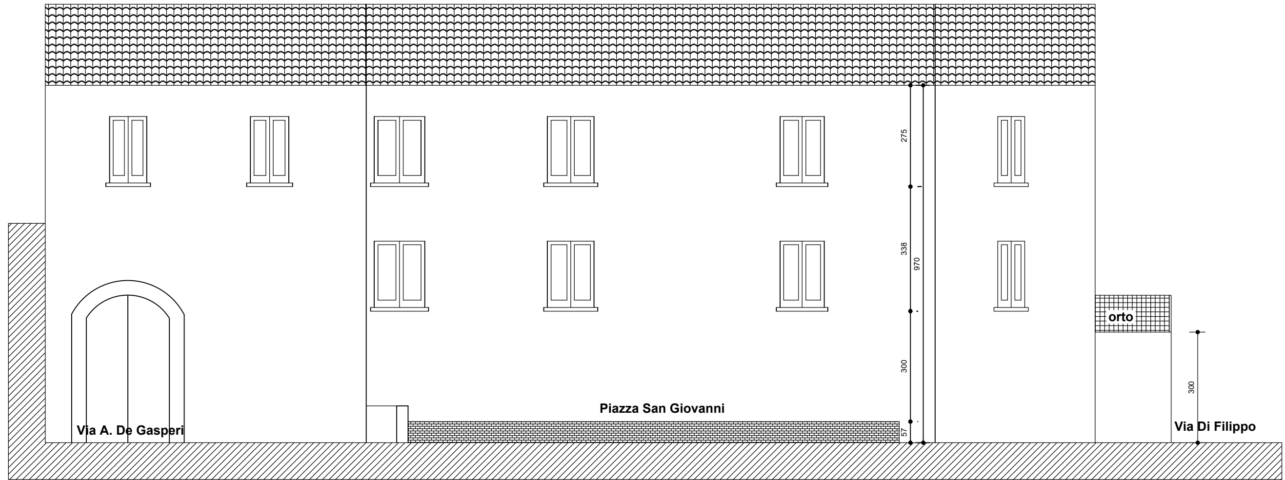
SEZIONE AA SU VIA DE GASPERI
