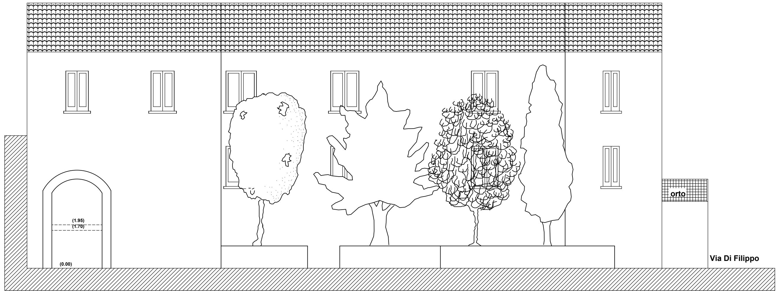
PROSPETTO SU VIA DE GASPERI
