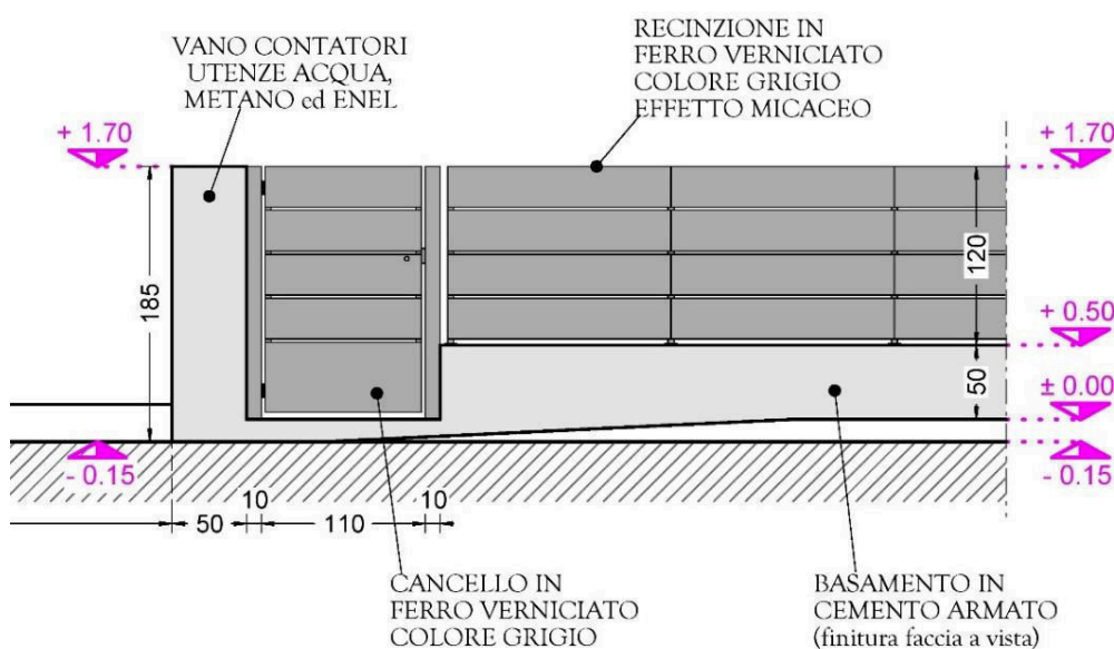
PARTICOLARE COSTRUTTIVO TIPO
