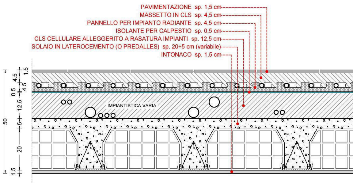
PARTICOLARE COSTRUTTIVO TIPO
