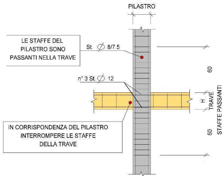
PARTICOLARE COSTRUTTIVO TIPO
