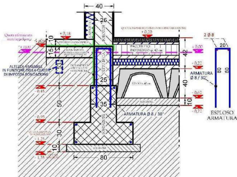
PARTICOLARE COSTRUTTIVO TIPO
