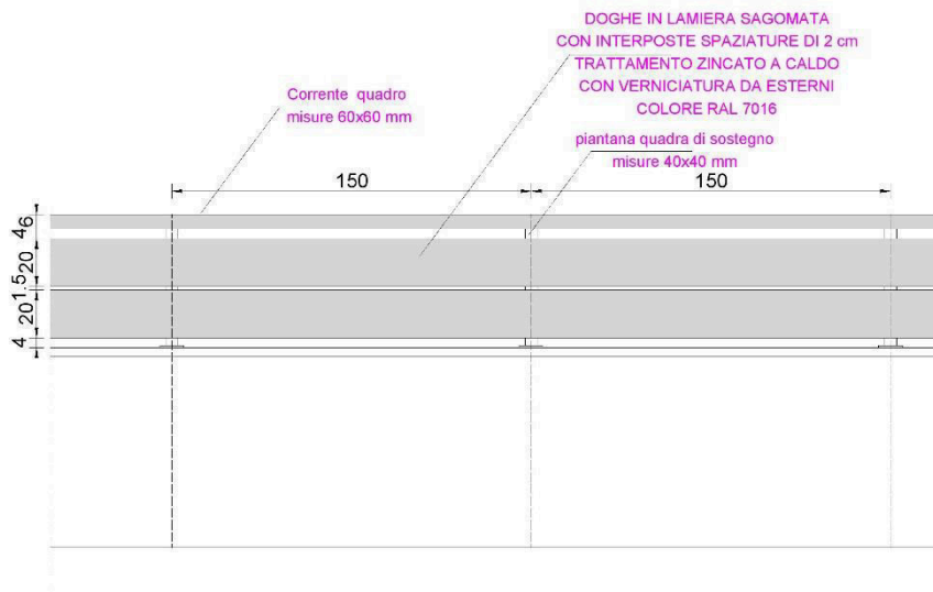
PARTICOLARE COSTRUTTIVO TIPO
