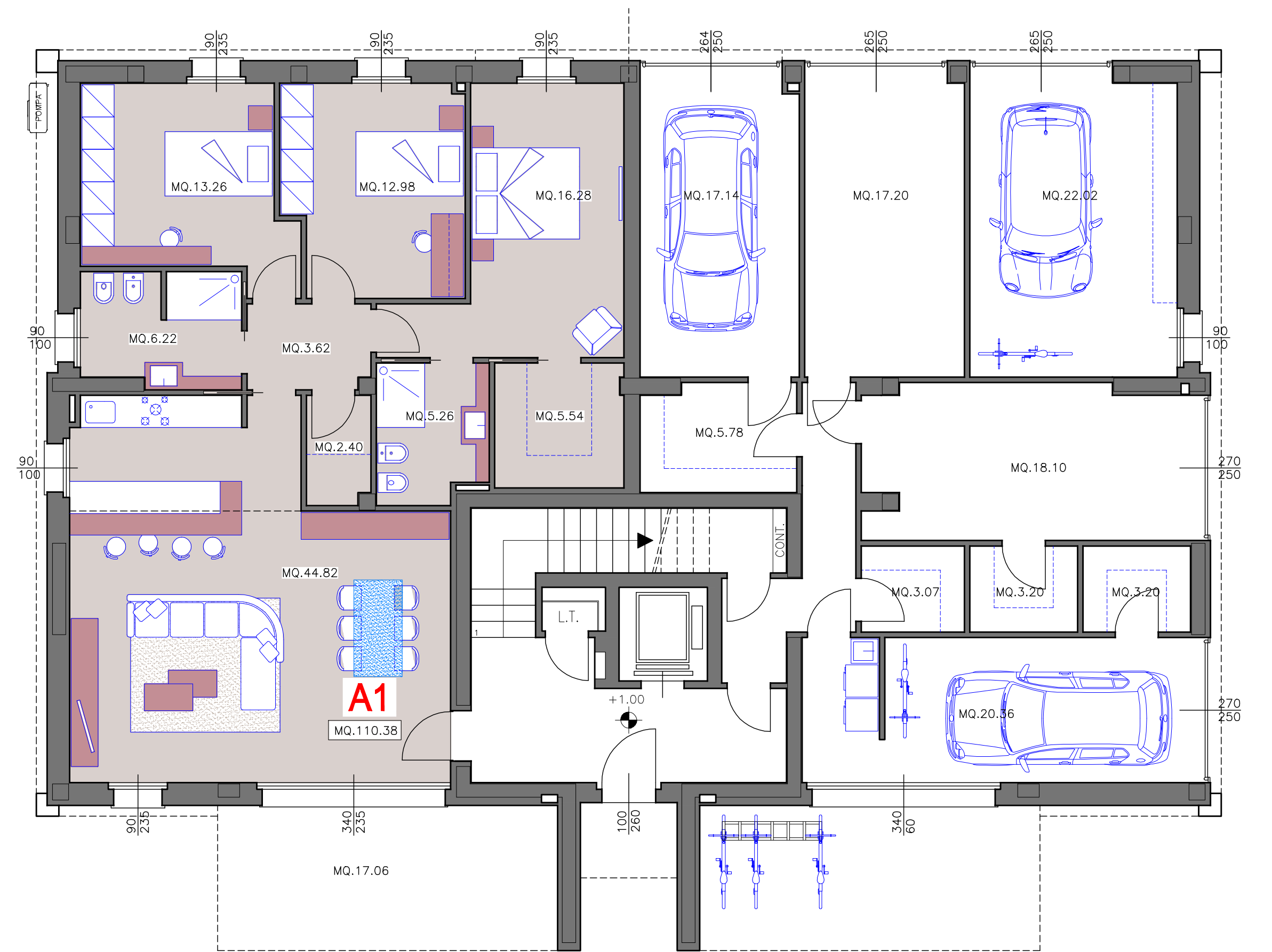
PIANO TERRA - variante B H=270
