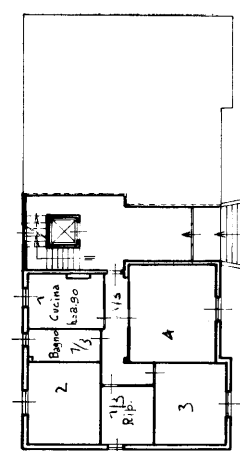
Pianta piano rialzato
