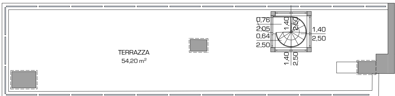
PIANTA PIANO OTTAVO
