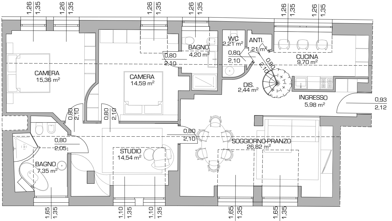
PIANTA PIANO SETTIMO
