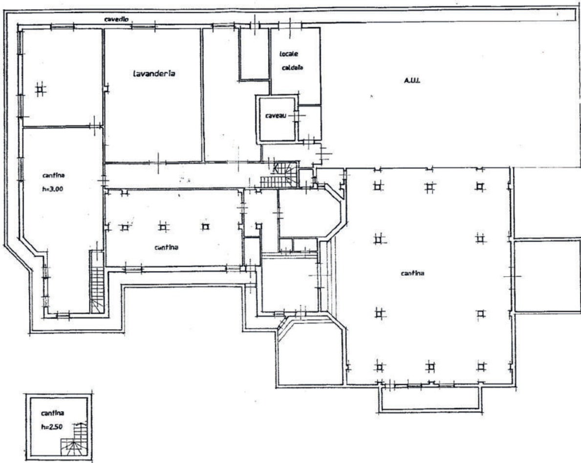
PIANO INTERRATO SECONDO
