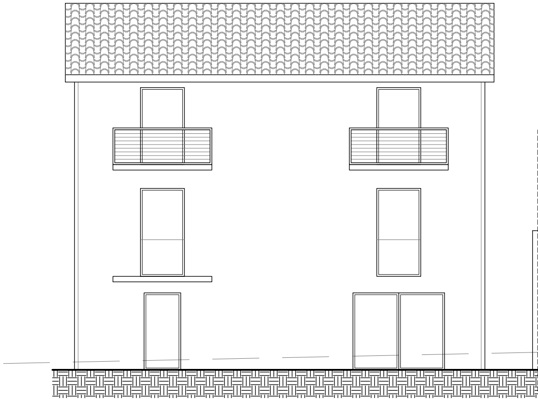
PROSPETTO OVEST
