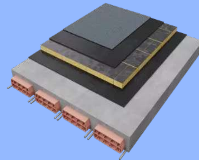
Figura 16 – Pacchetto copertura
