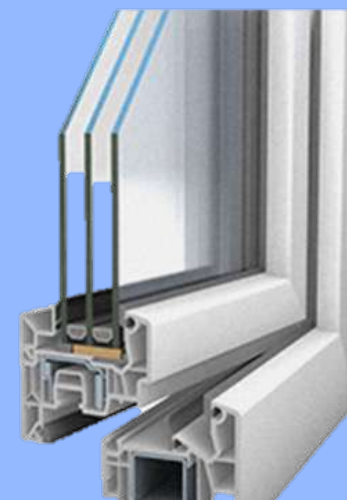
Figura 29 – Serramento PVC
