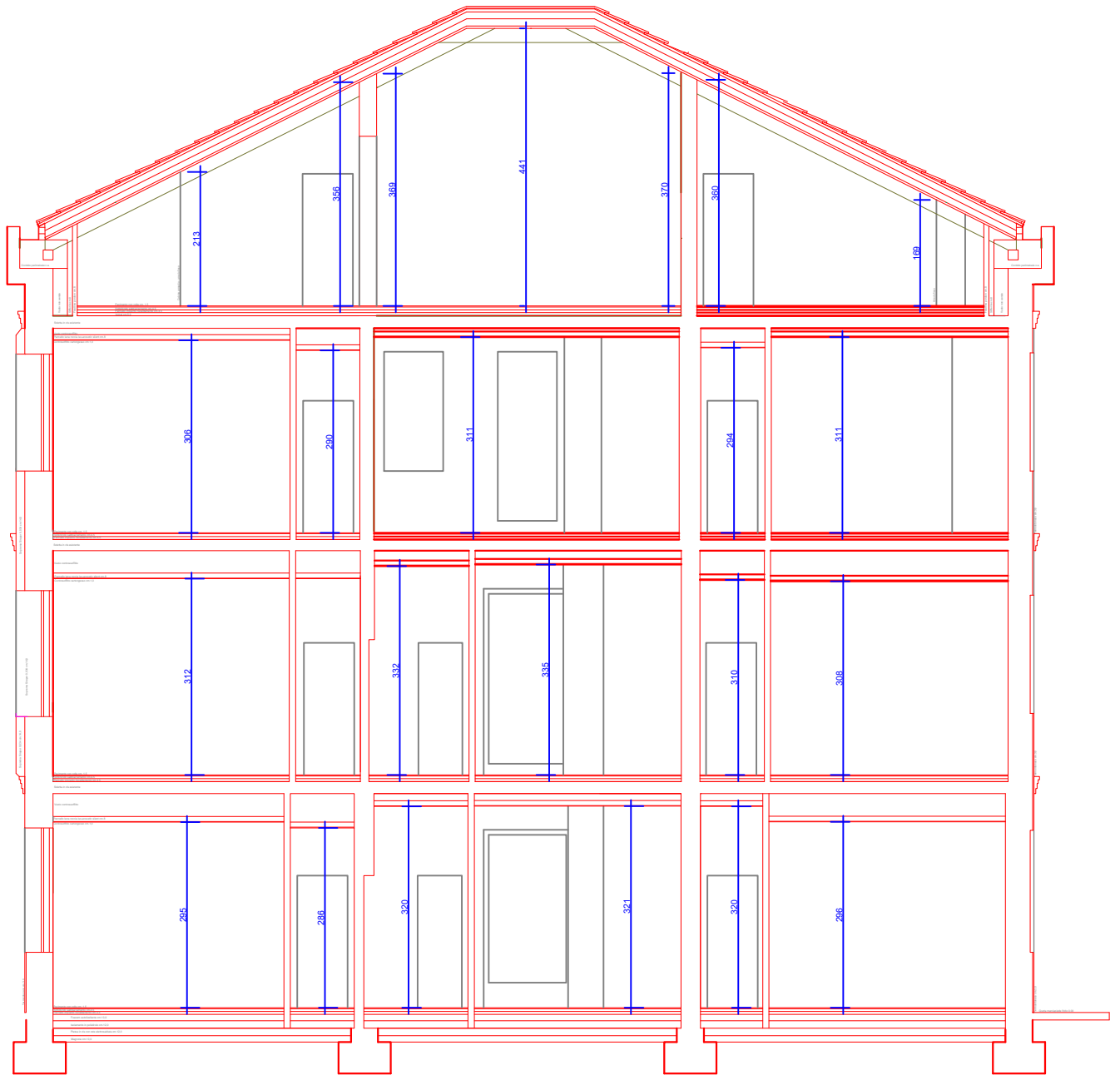
SEZIONE A-A
