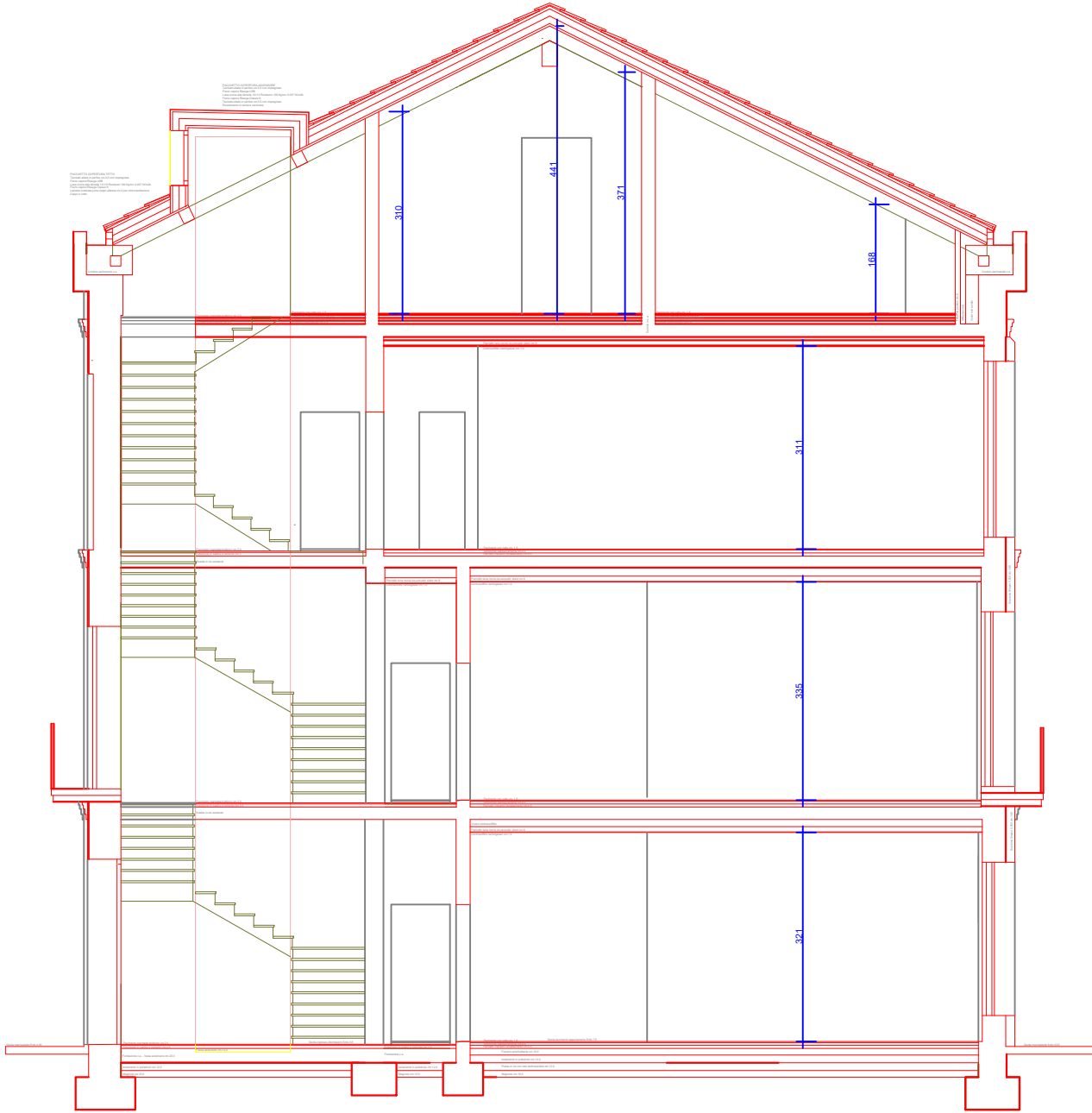
SEZIONE B-B
