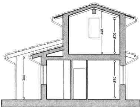
Sezione B-B
