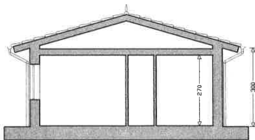
Sezione A-A
