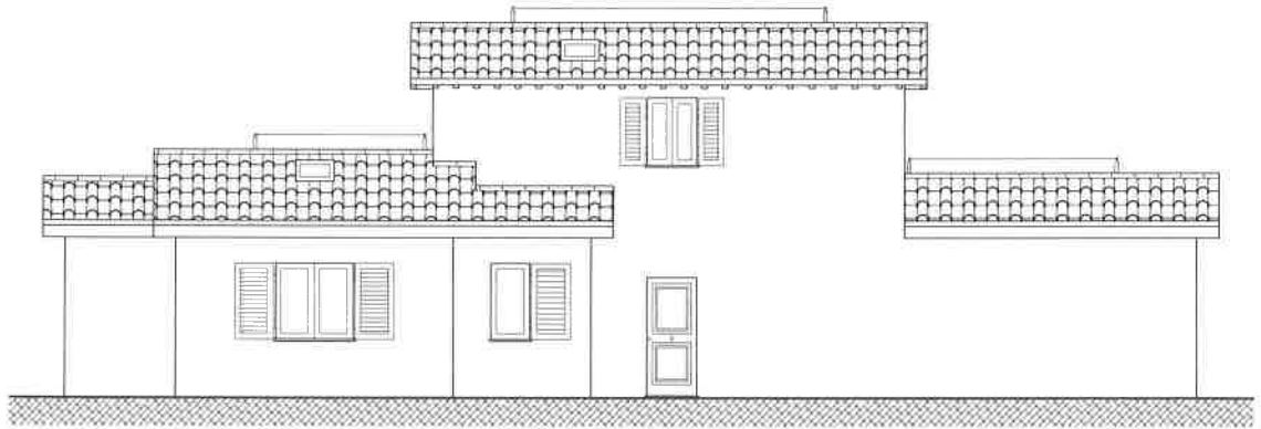
Prospetto Est
