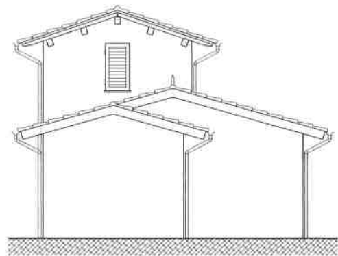
Prospetto Sud
