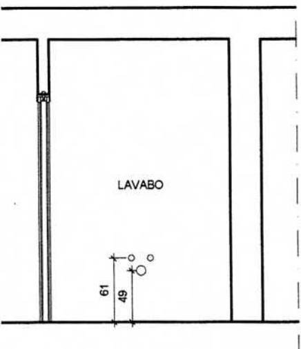
SEZIONE AA
