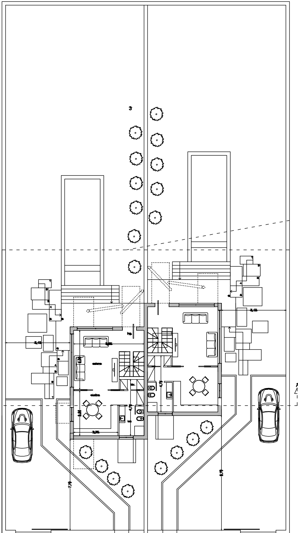
PIANTA PIANO TERRA Scale 1:100
