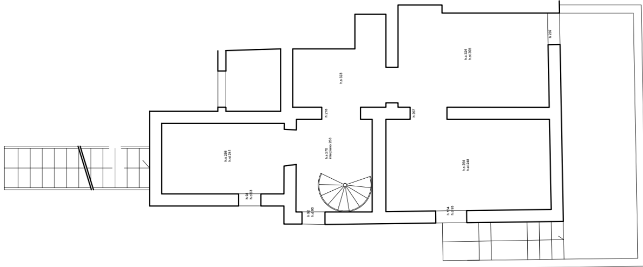
PIANTA PIANO TERRA 1:100
