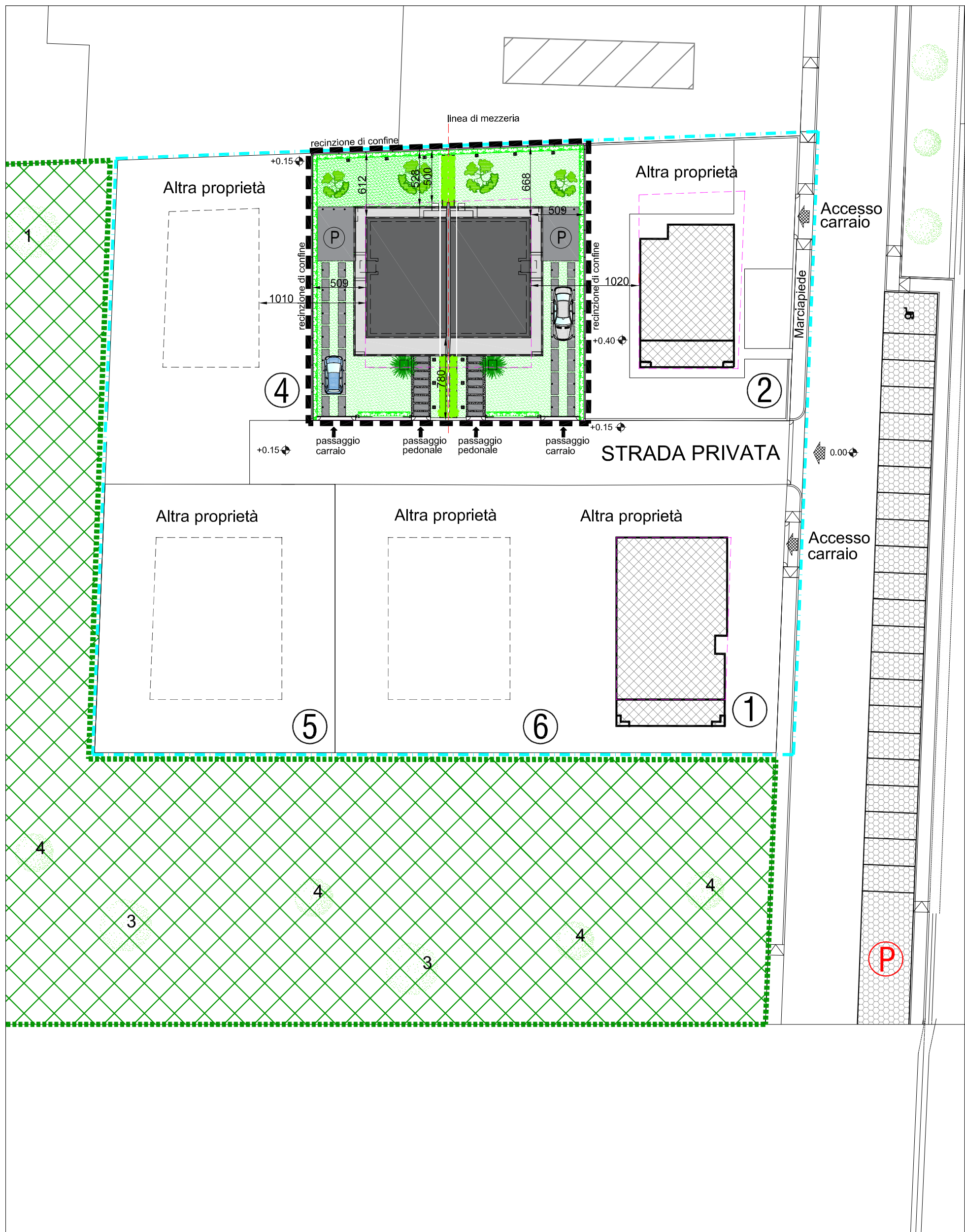
PLANIMETRIA GENERALE STATO DI PROGETTO SCALA 1:500
