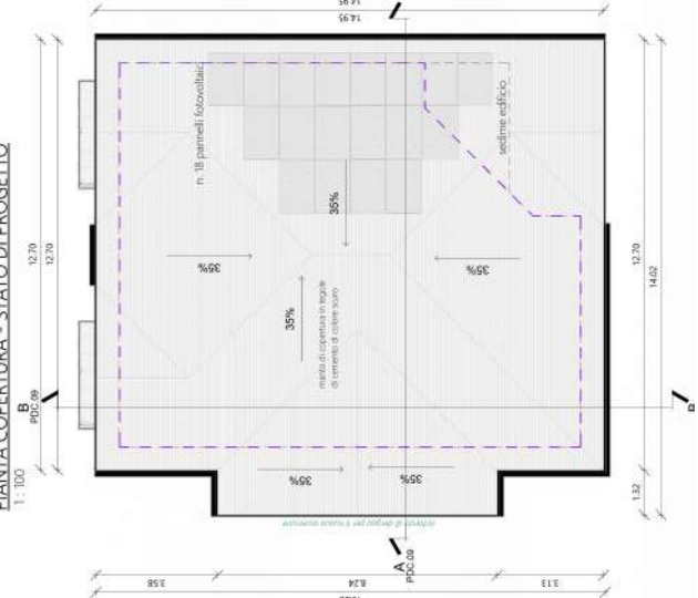
PIANTA COPERTURA - STATO DI PROGETTO
