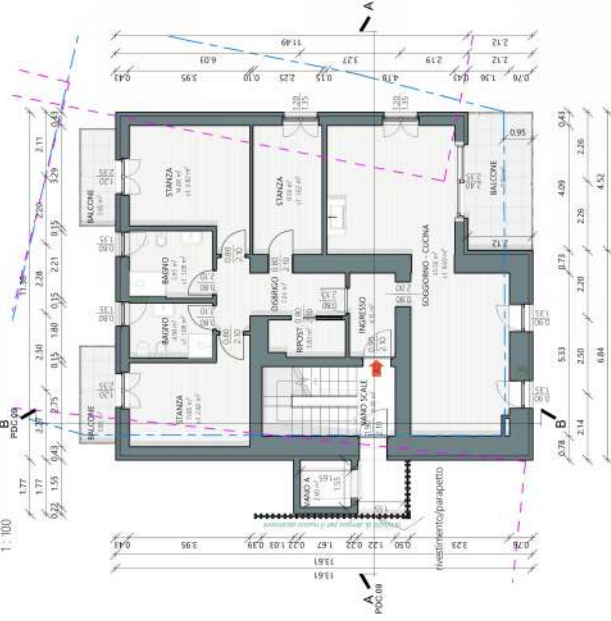
PIANO PRIMO - STATO DI PROGETTO
