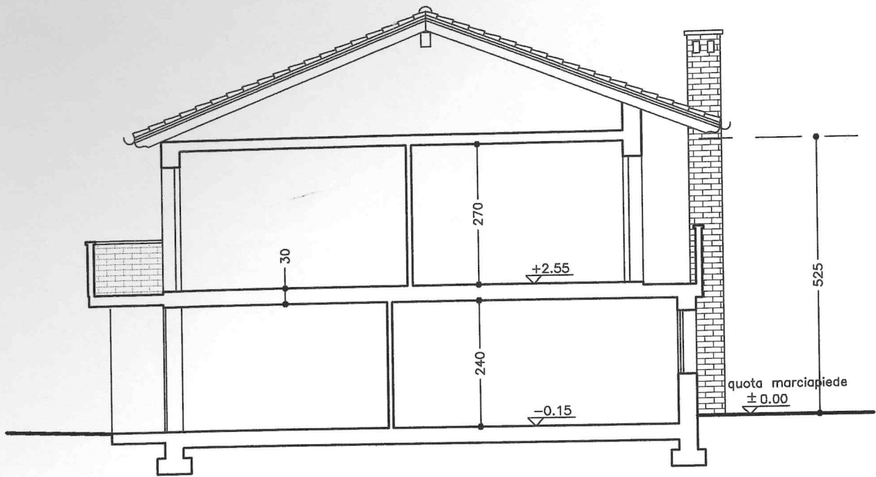
SEZIONE A-A
