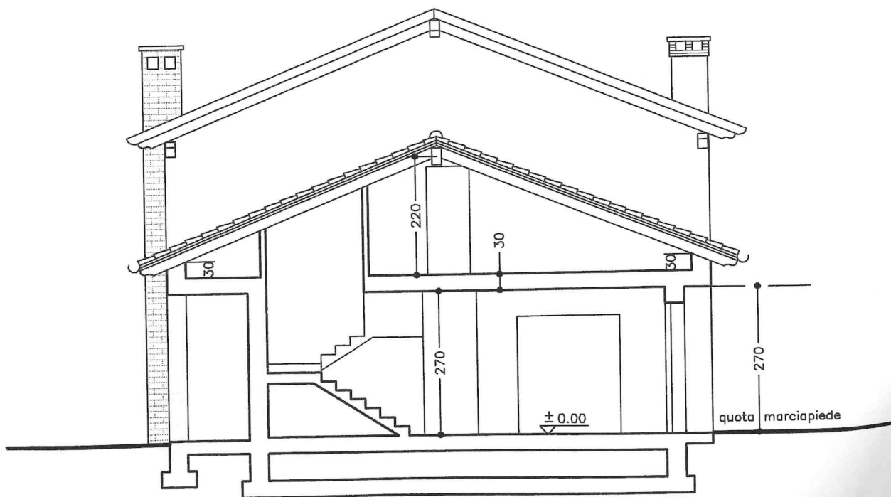
SEZIONE B-B
